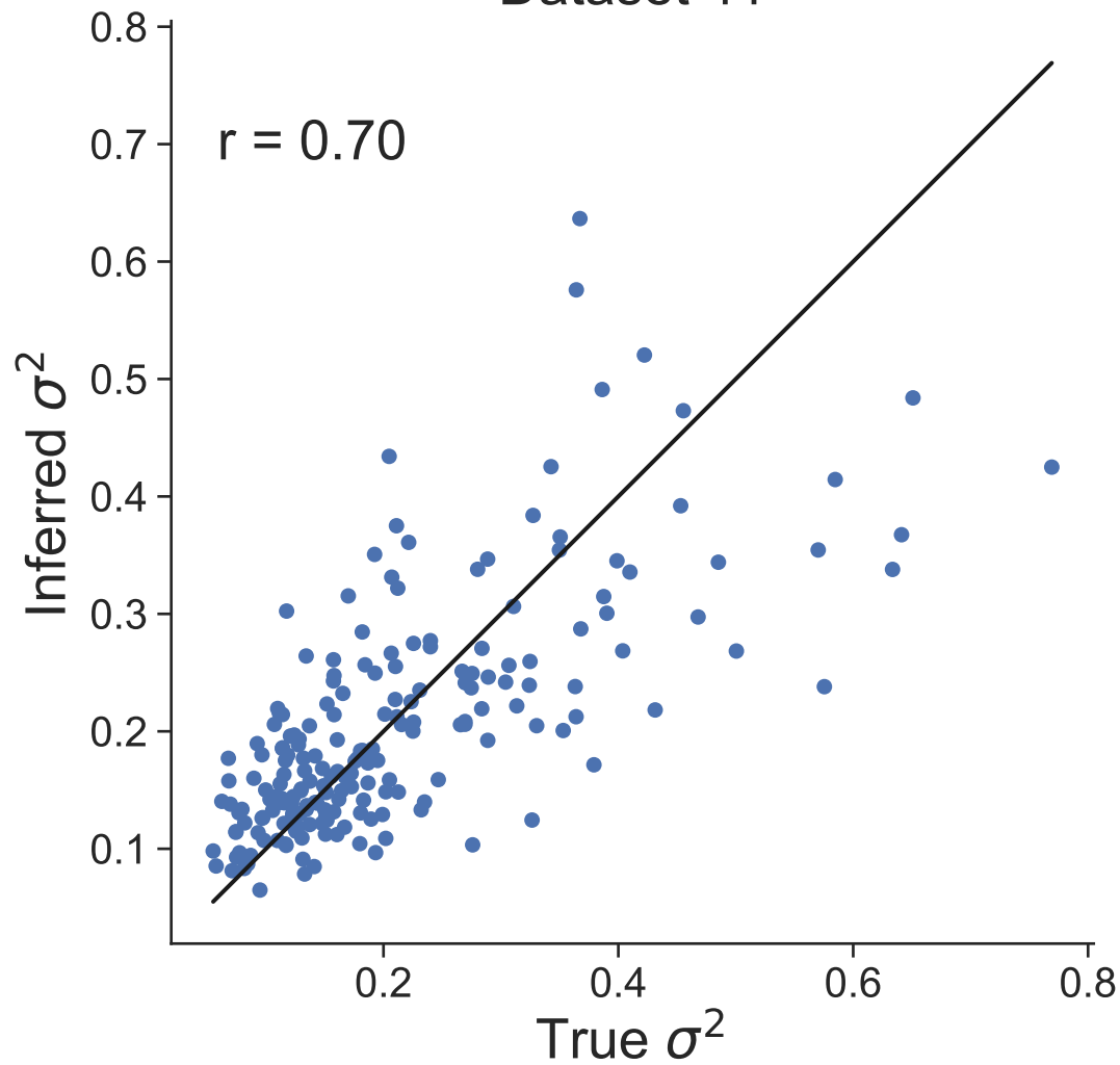
Dataset 41
