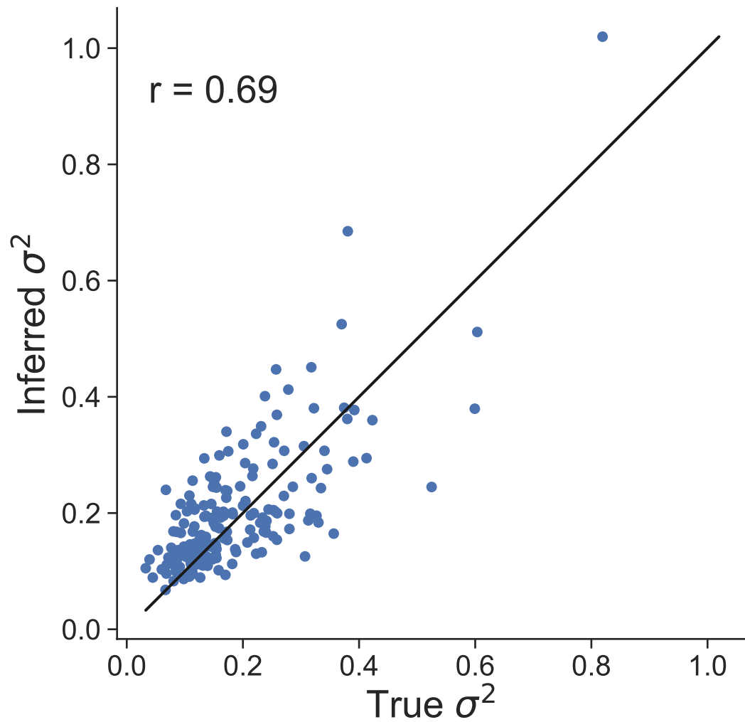
Dataset 48
