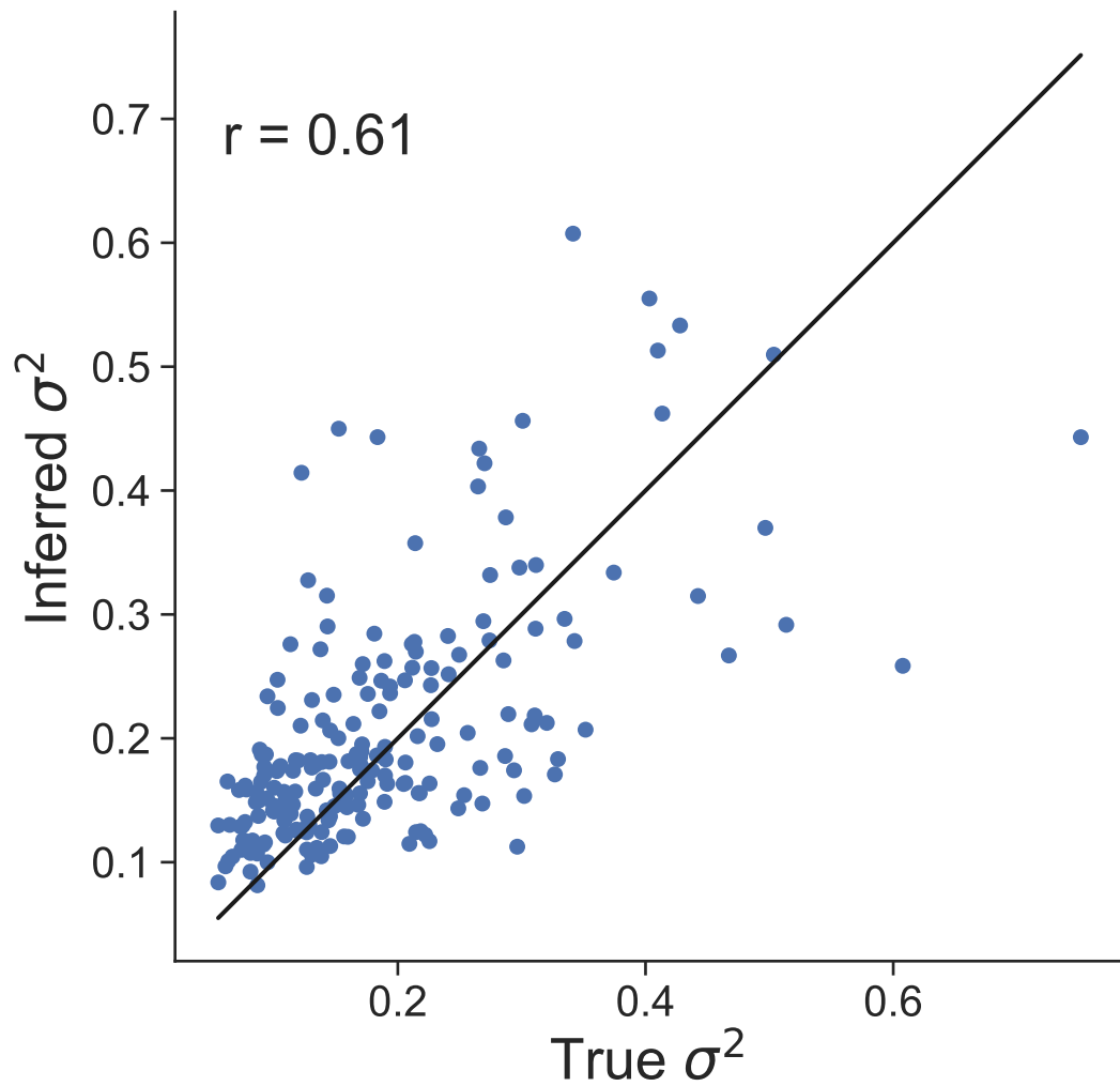
Dataset 23
