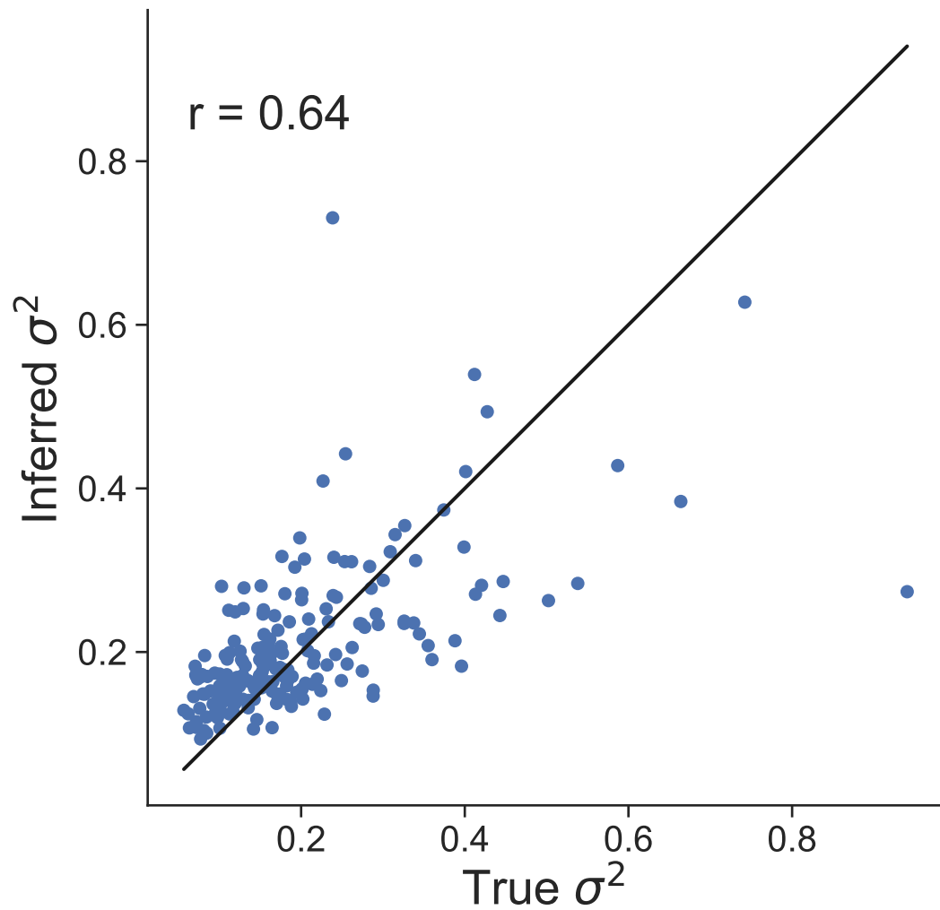
Dataset 21
