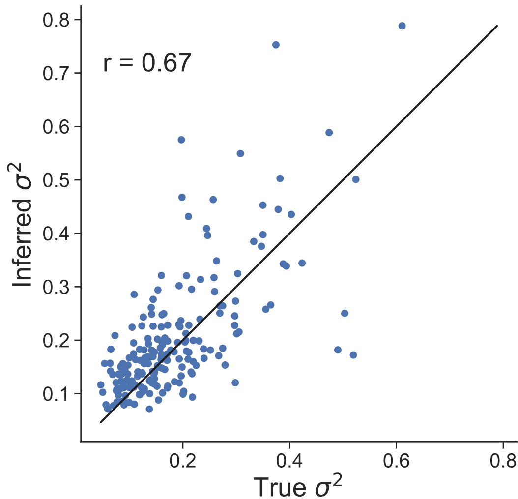
Dataset 25
