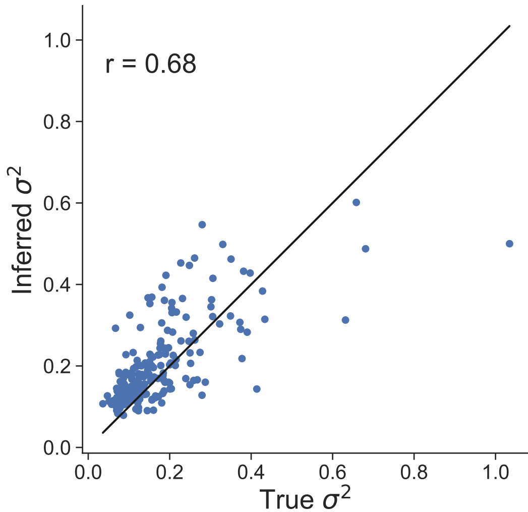
Dataset 31
