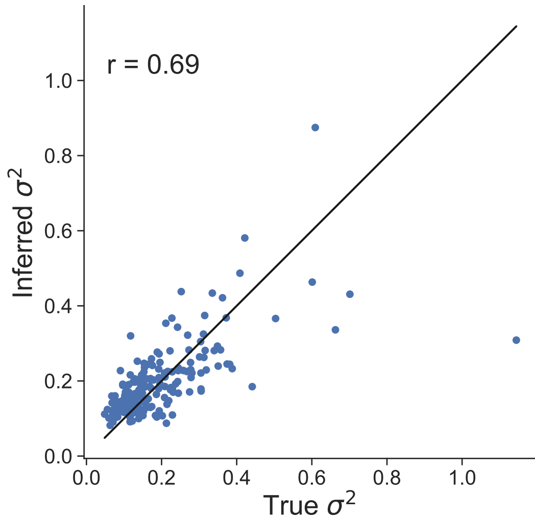
Dataset 18
