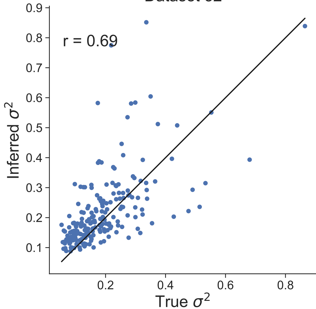
Dataset 32
