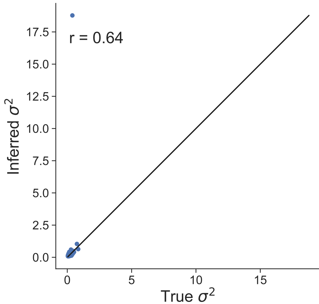
Dataset 14
