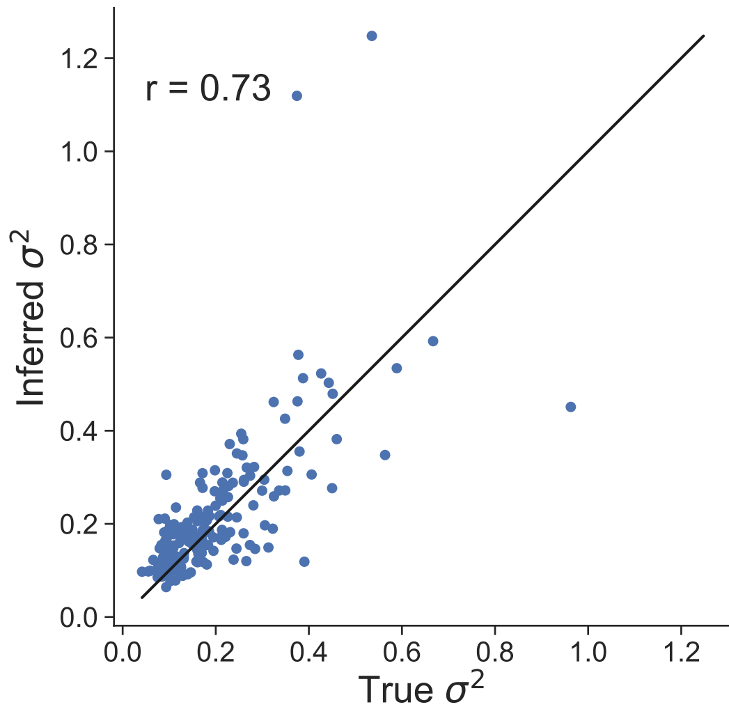
Dataset 24
