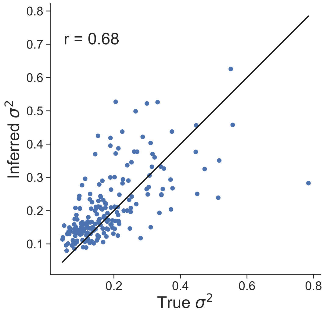
Dataset 35
