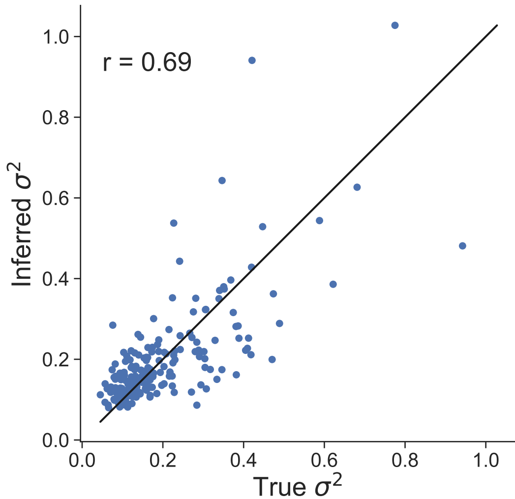
Dataset 29
