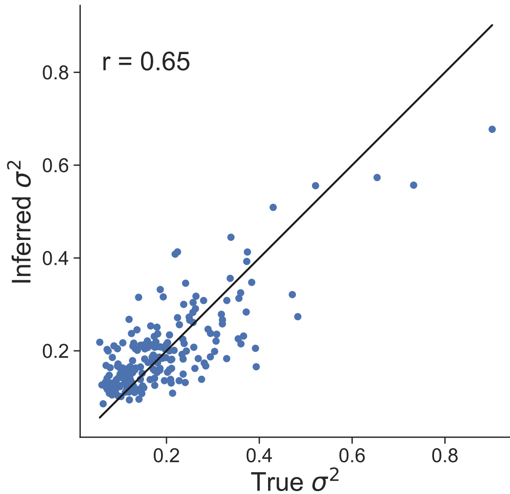
Dataset 43
