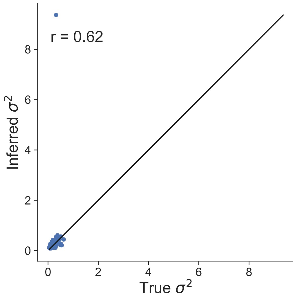
Dataset 39
