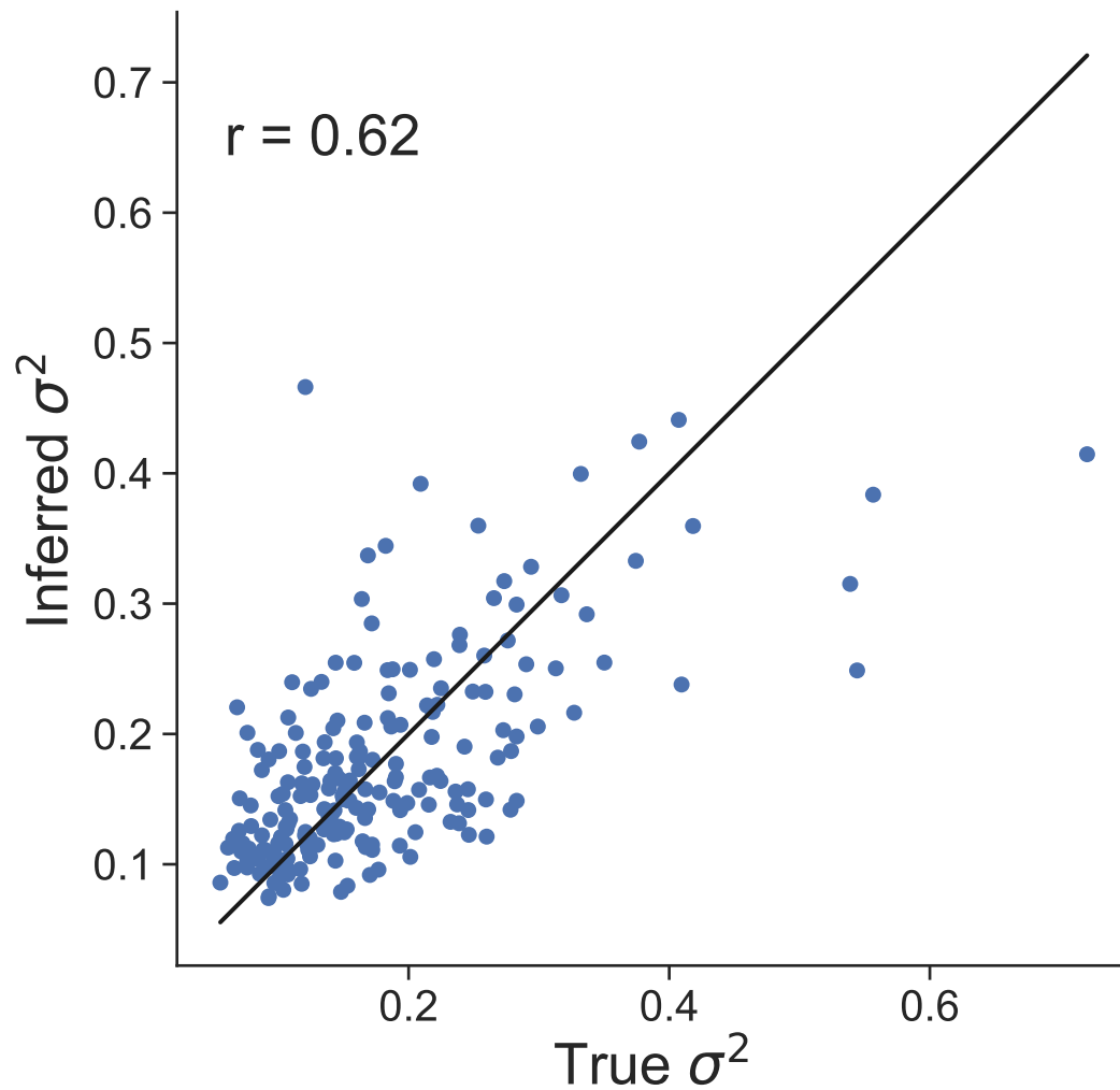
Dataset 45
