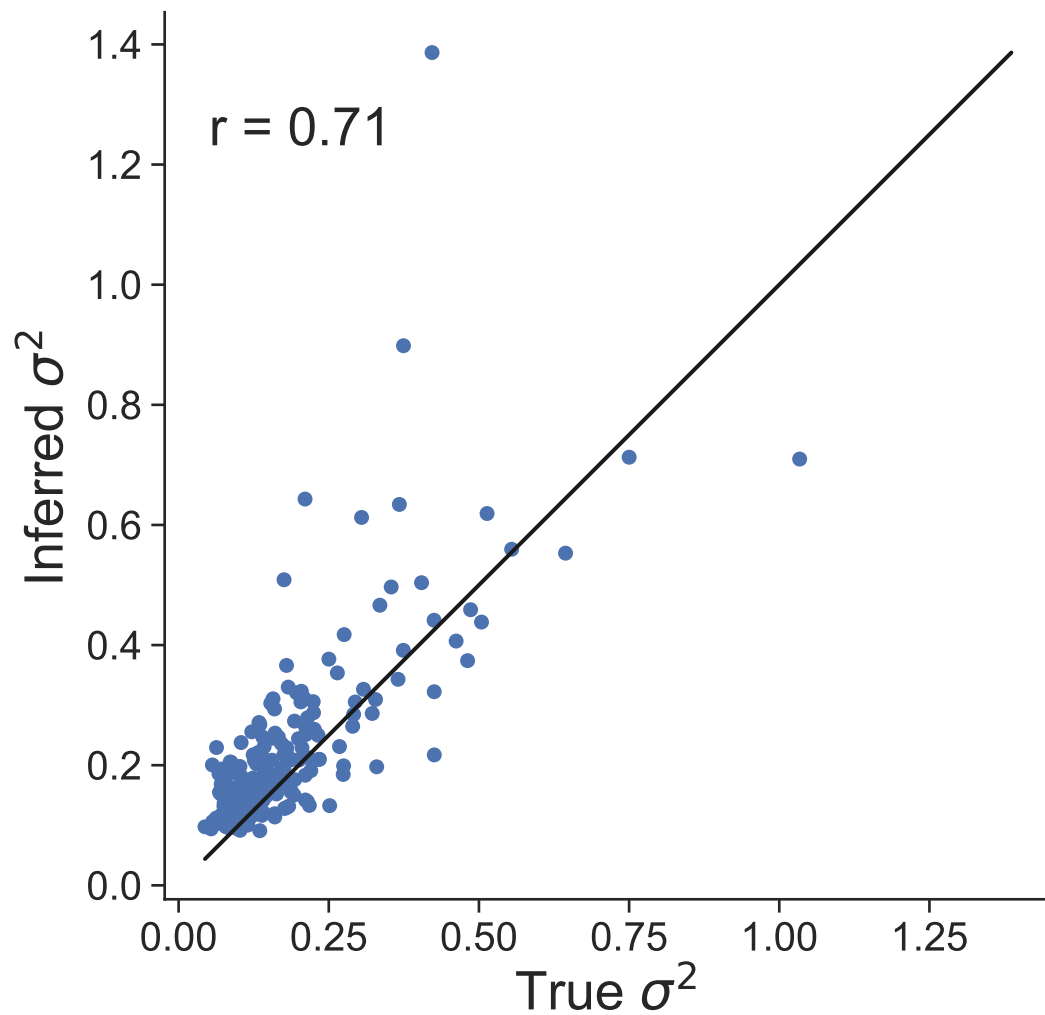
Dataset 0
