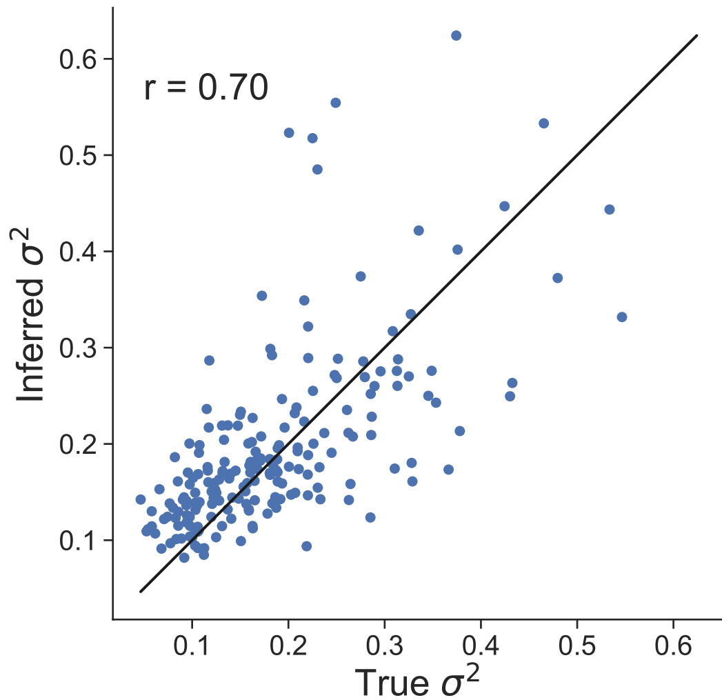
Dataset 47
