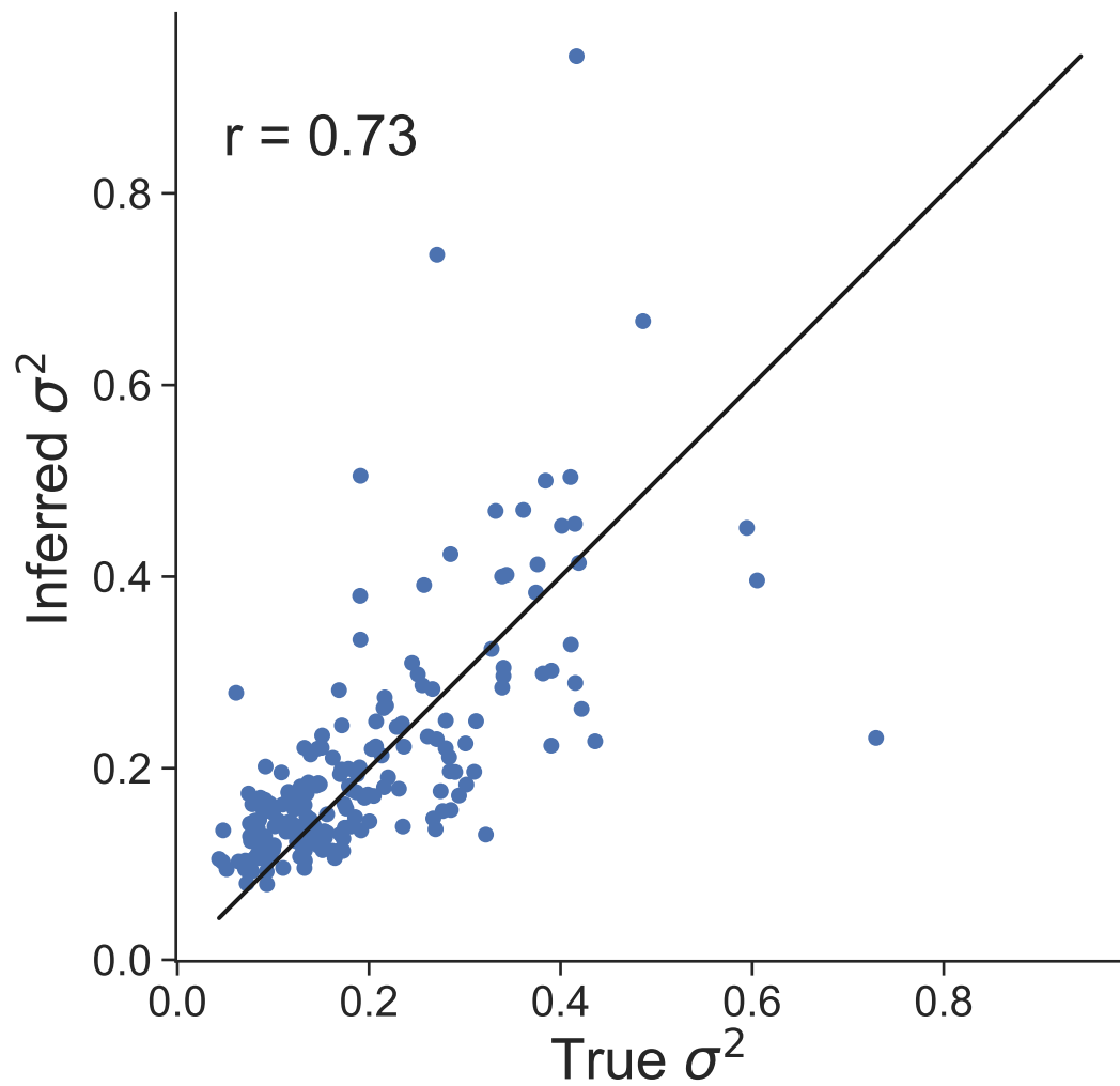
Dataset 26
