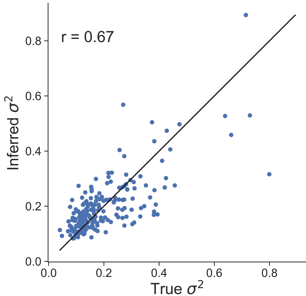
Dataset 27
