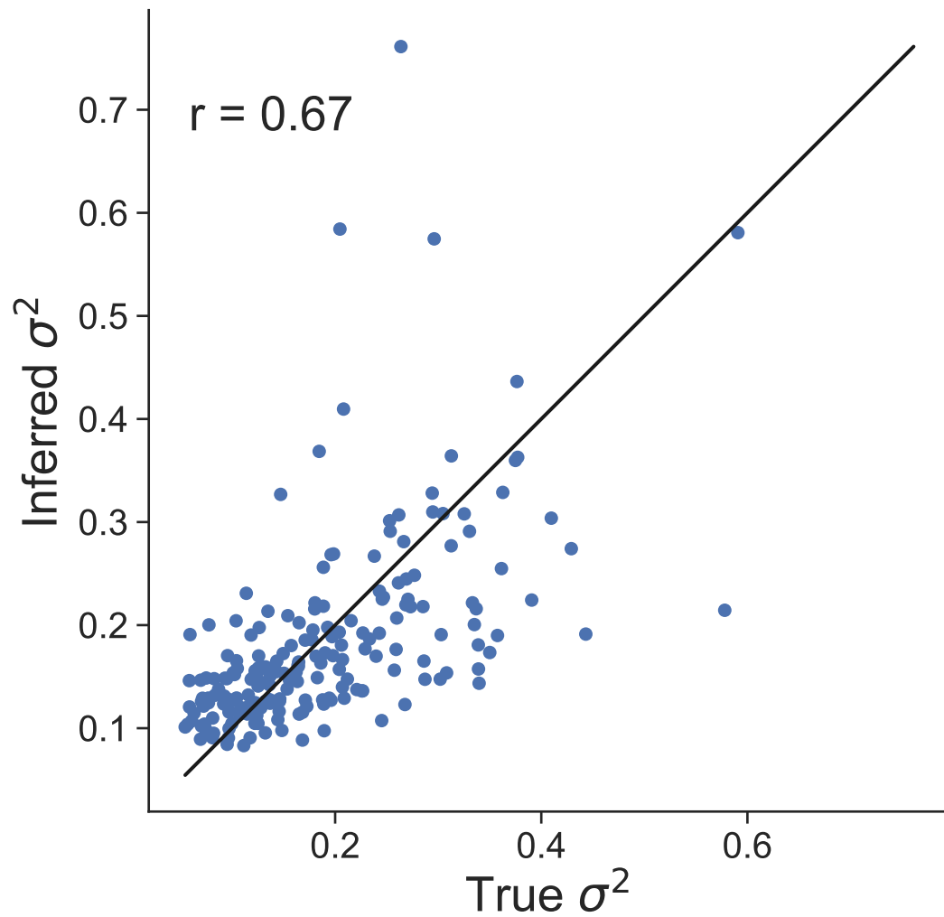
Dataset 38
