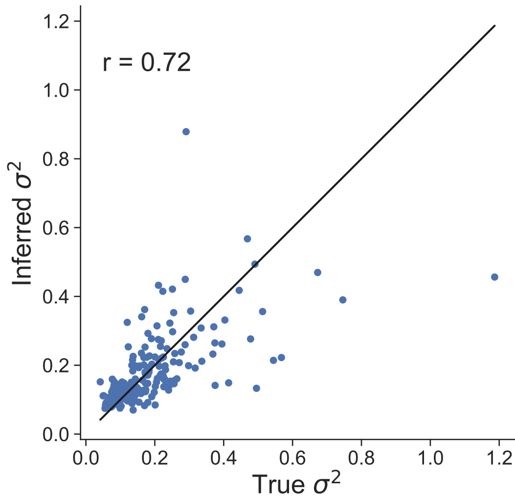
Dataset 42
