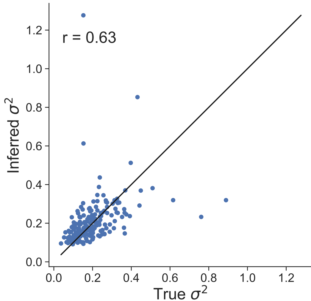
Dataset 12
