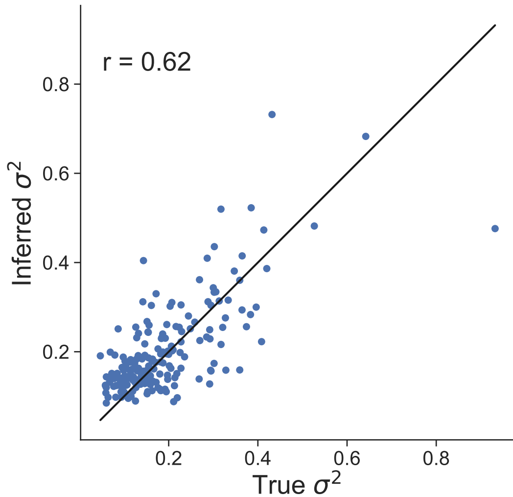
Dataset 8
