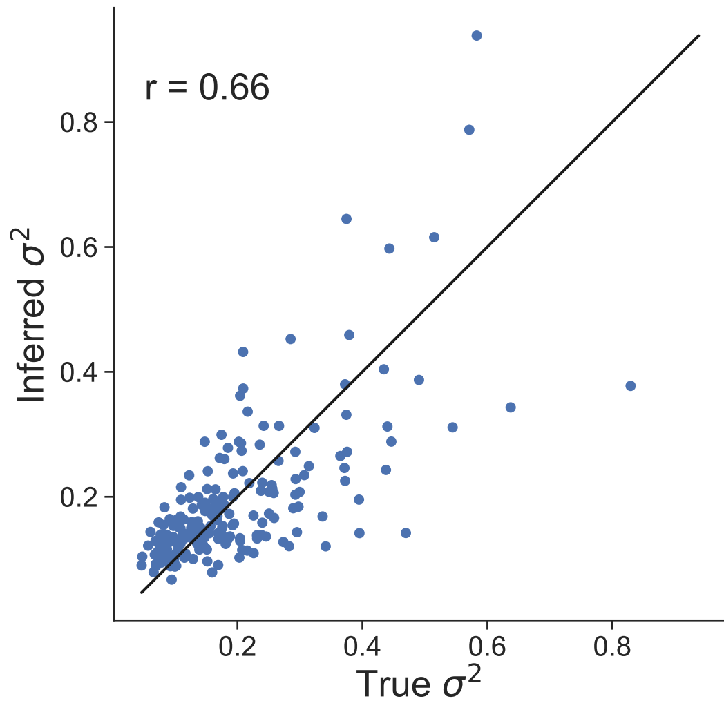
Dataset 6
