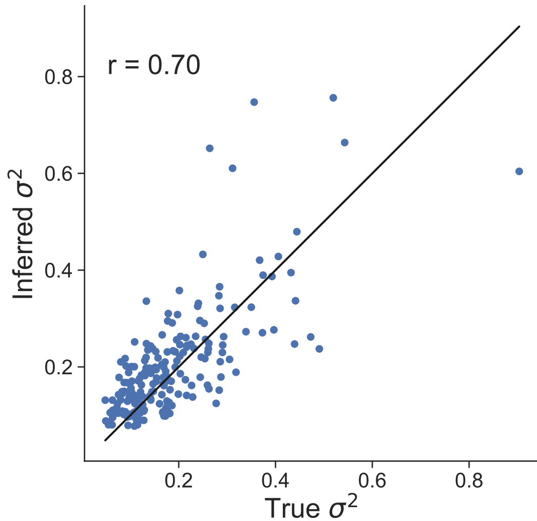
Dataset 20
