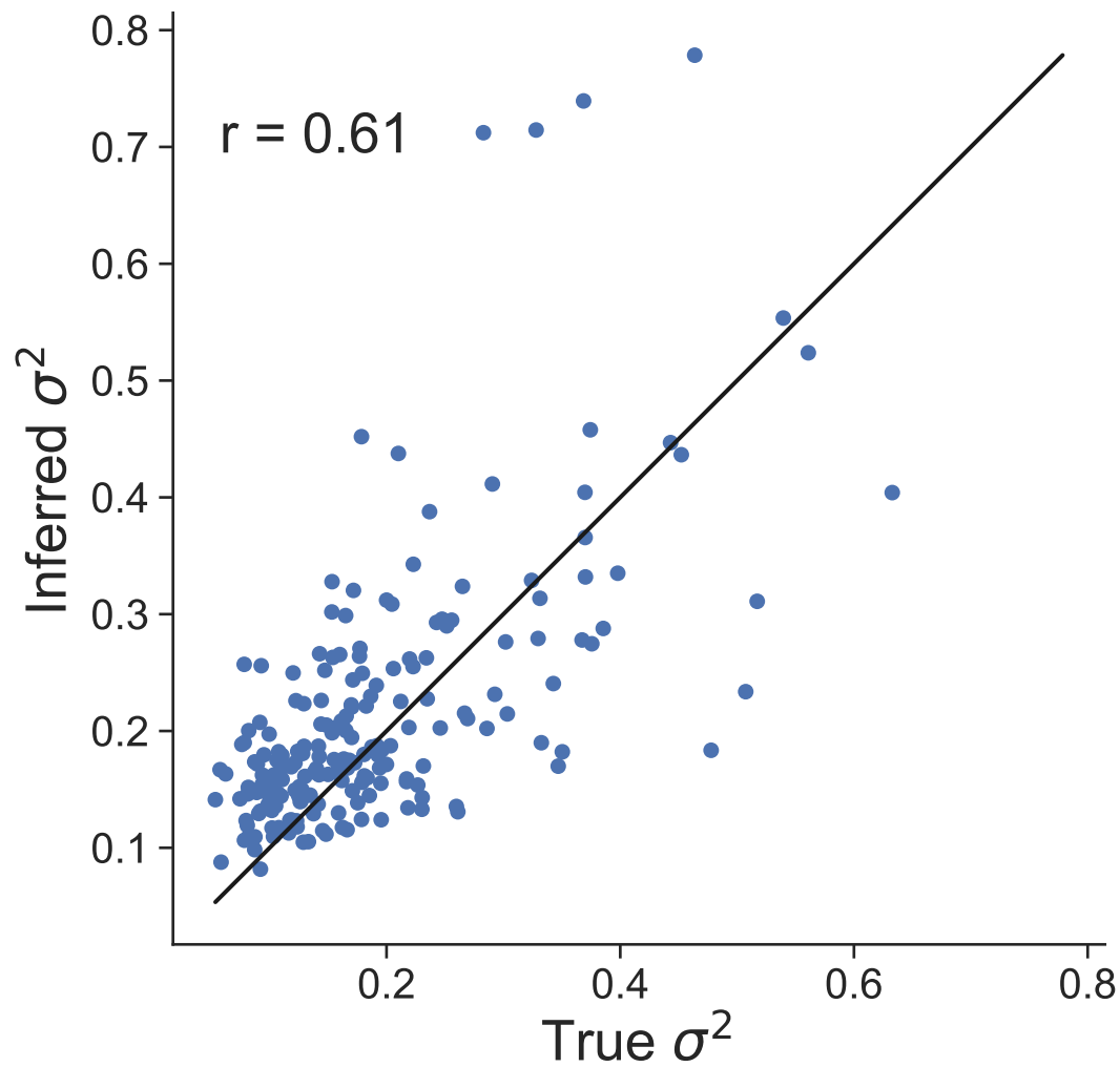
Dataset 17
