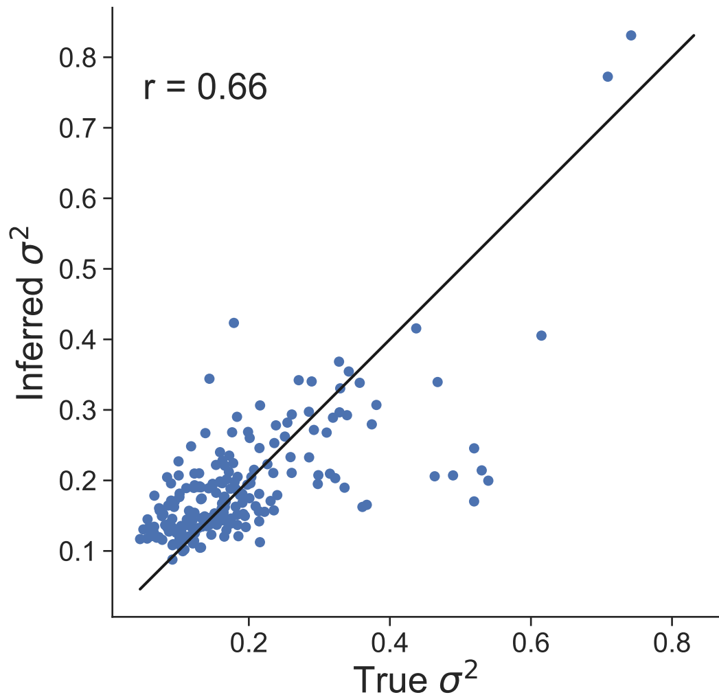
Dataset 28
